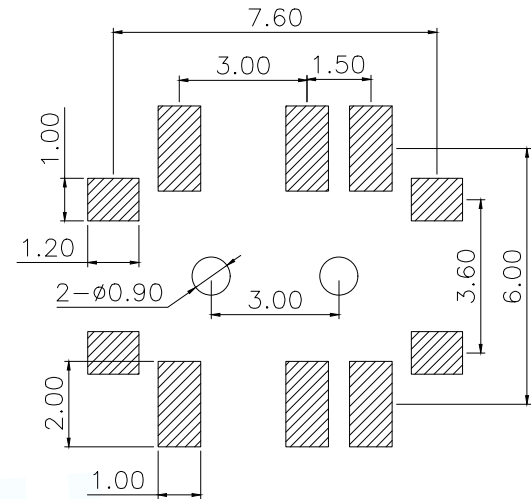
安装尺寸
