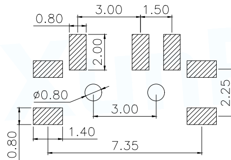
安装尺寸
