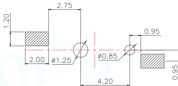
安装尺寸
