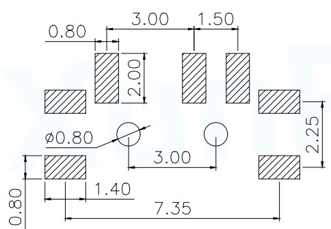
安装尺寸
