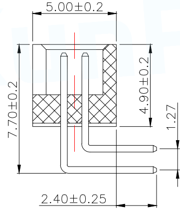
A-A SECTION
