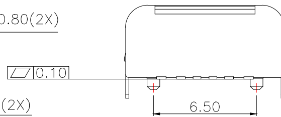
"E"向视图
