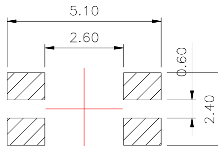
PCB.焊接图
