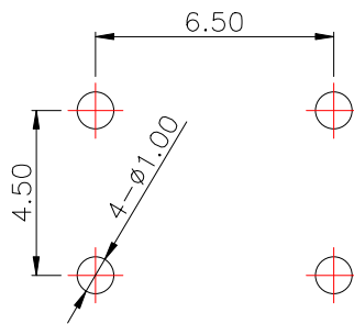
PCB.焊接图
