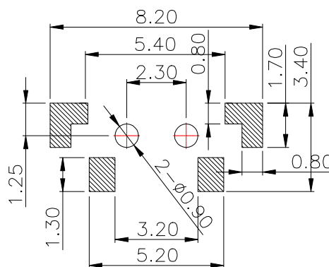
PCB.焊接图
